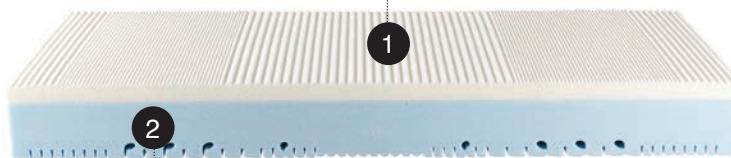
LASTRA IN AQUATERM SENZA CFC A 7 ZONE. SPESSORE 15 CM. DENSITA' 25 Kg.M3.KPA 3,8 SAGOMATURA PER UN PERFETTO ALLINEAMENTO VERTEBRALE.
